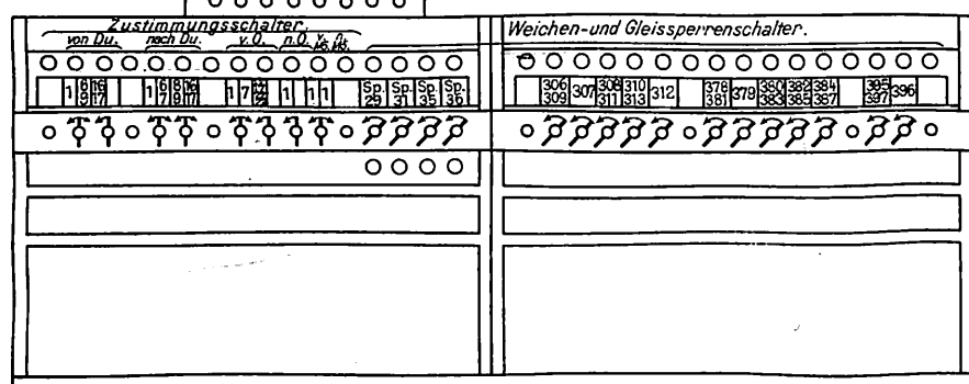
Abb. 2. Stellwerk XI.
