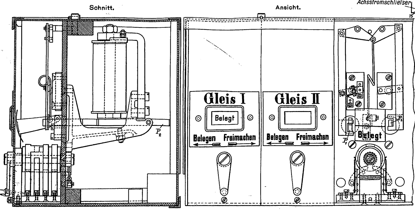
Abb. 5. Belegt-Einrichtung.
