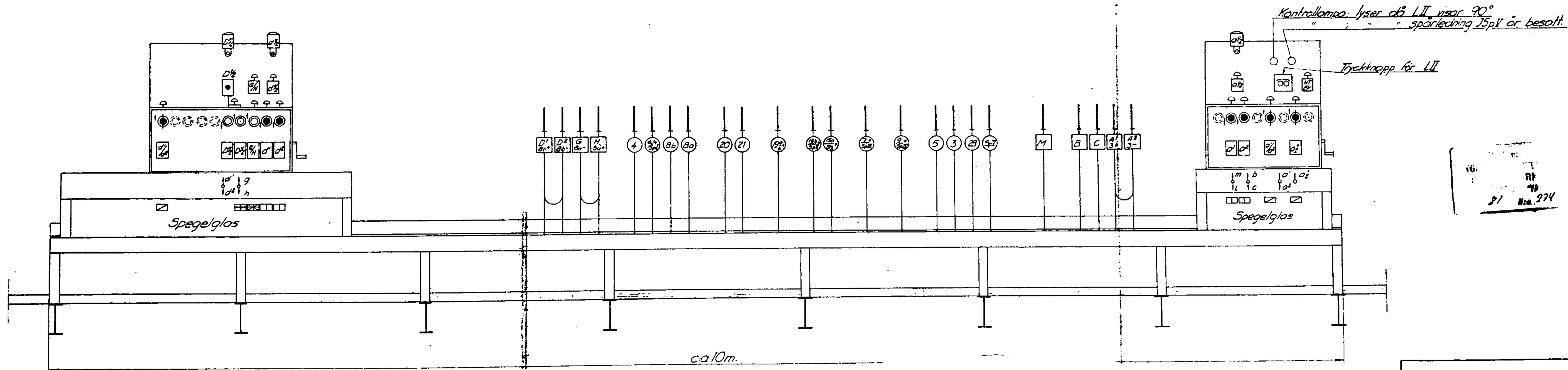
Ställverk II 1:20
