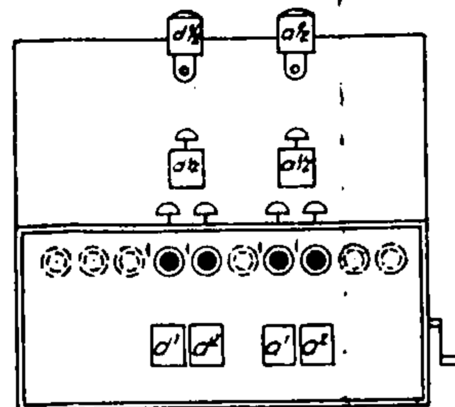
Stationsblockapparat. Skala 1:20
