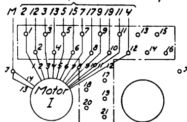
Klämmor på kontaktplintar
