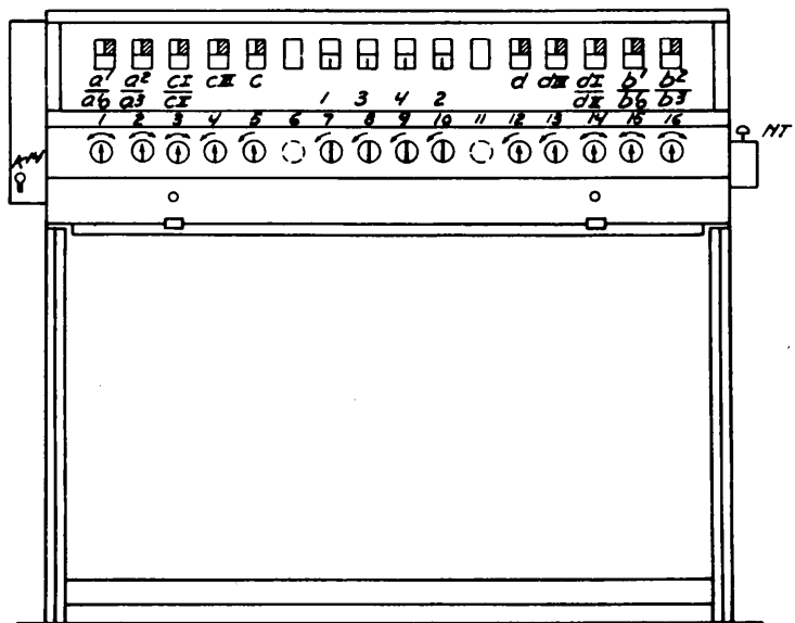
Ställverk
