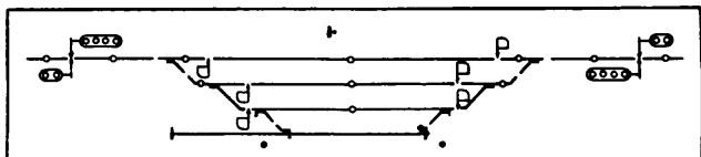
Illuminerad spårplan
