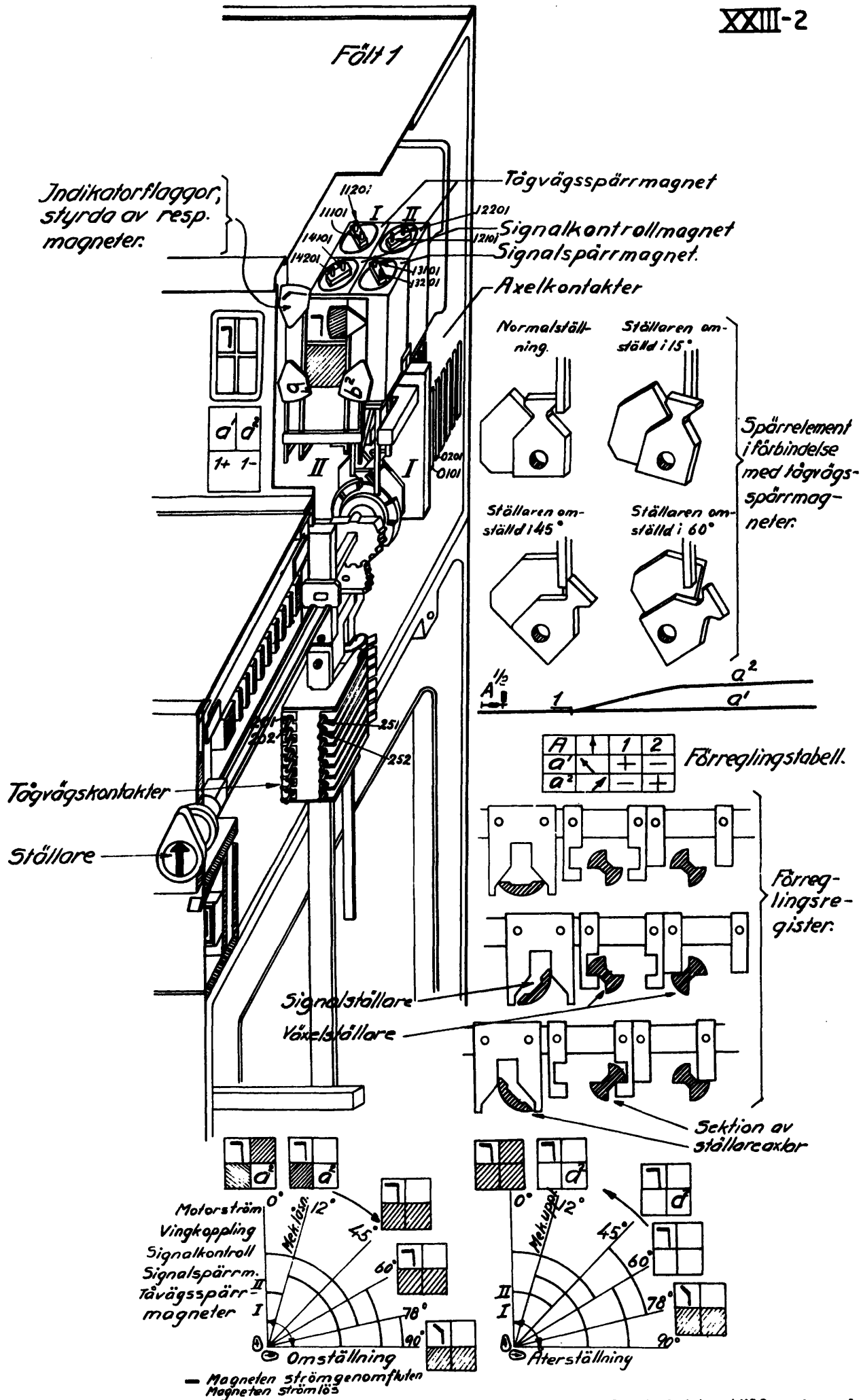
Elektriskt ställverk med mekaniskt register. TÄGVÄGSSIGNALSTÄLLARE.
