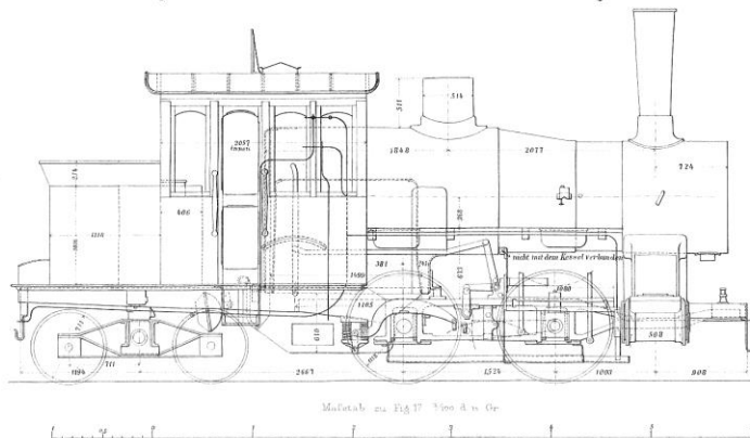
Fig. 17. Verbund-Lokomotive der Lake-Street-Hochbahn in Chicago.
