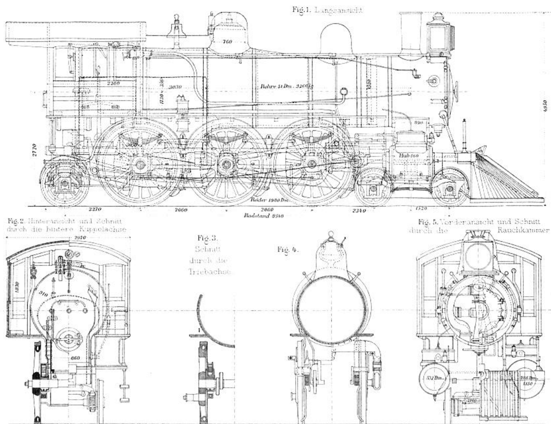
Fig. 1. 5. Verbund-Personenzug-Locomotive der Chicago-Milwaukee- und St. Paul-Bahn. Erbaut von den Rhode Island Locomotive Works in Providence.
