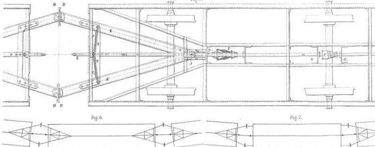
Fig. 1-7. Doppeltragsbrücke für Eisenbahnfahrzeuge. Bauart Lentz.
