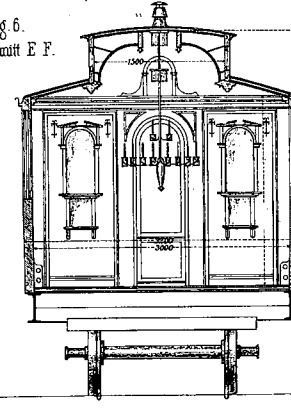
Fig. 7. Stirnansicht des Speisewagens.
