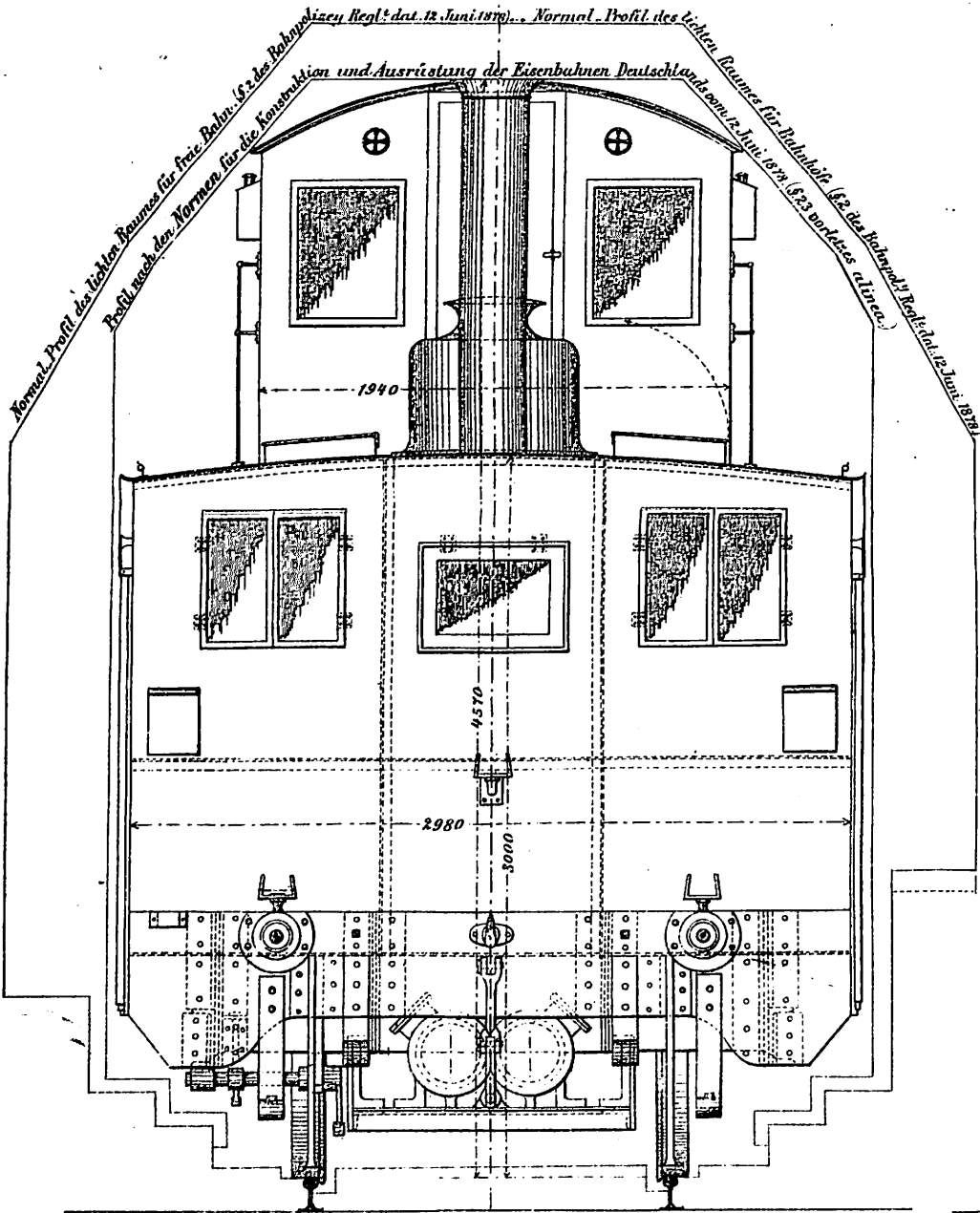
Vorder-Ansicht.
