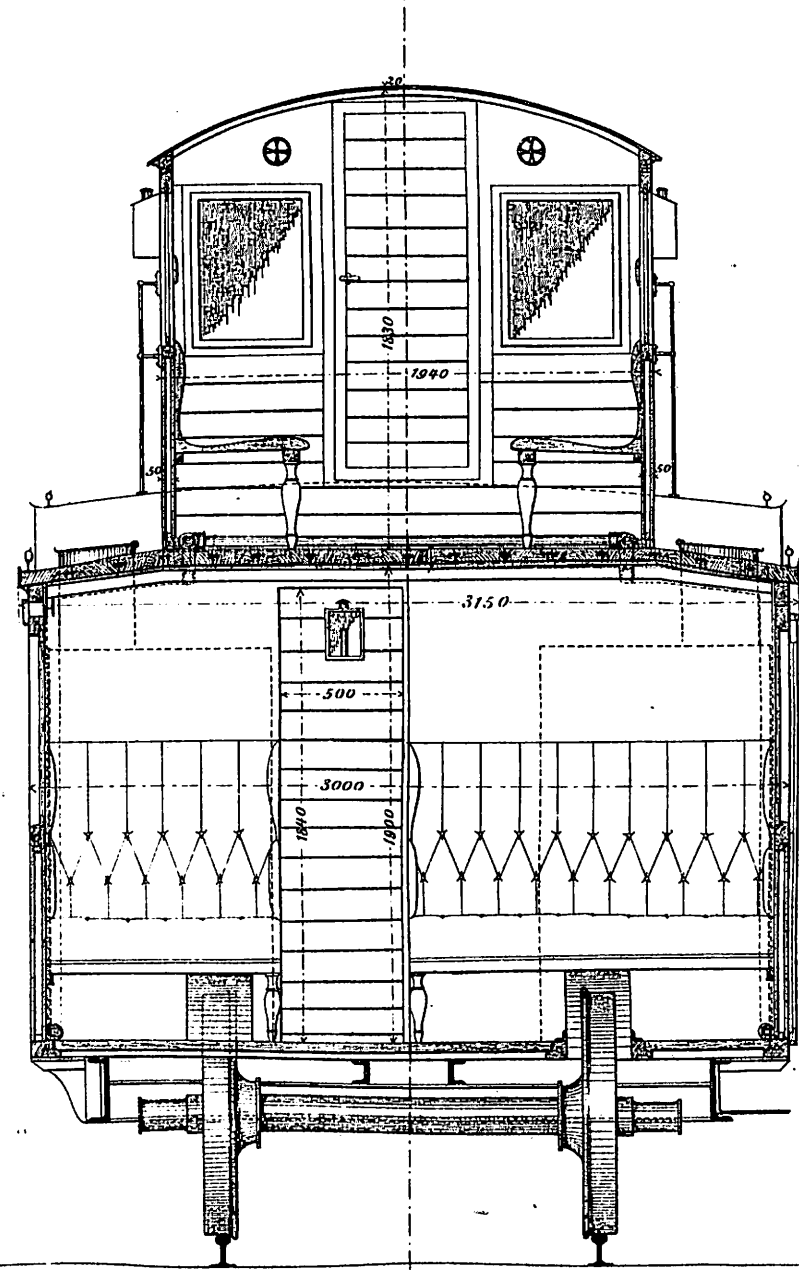
Schnitt CD, EF.
