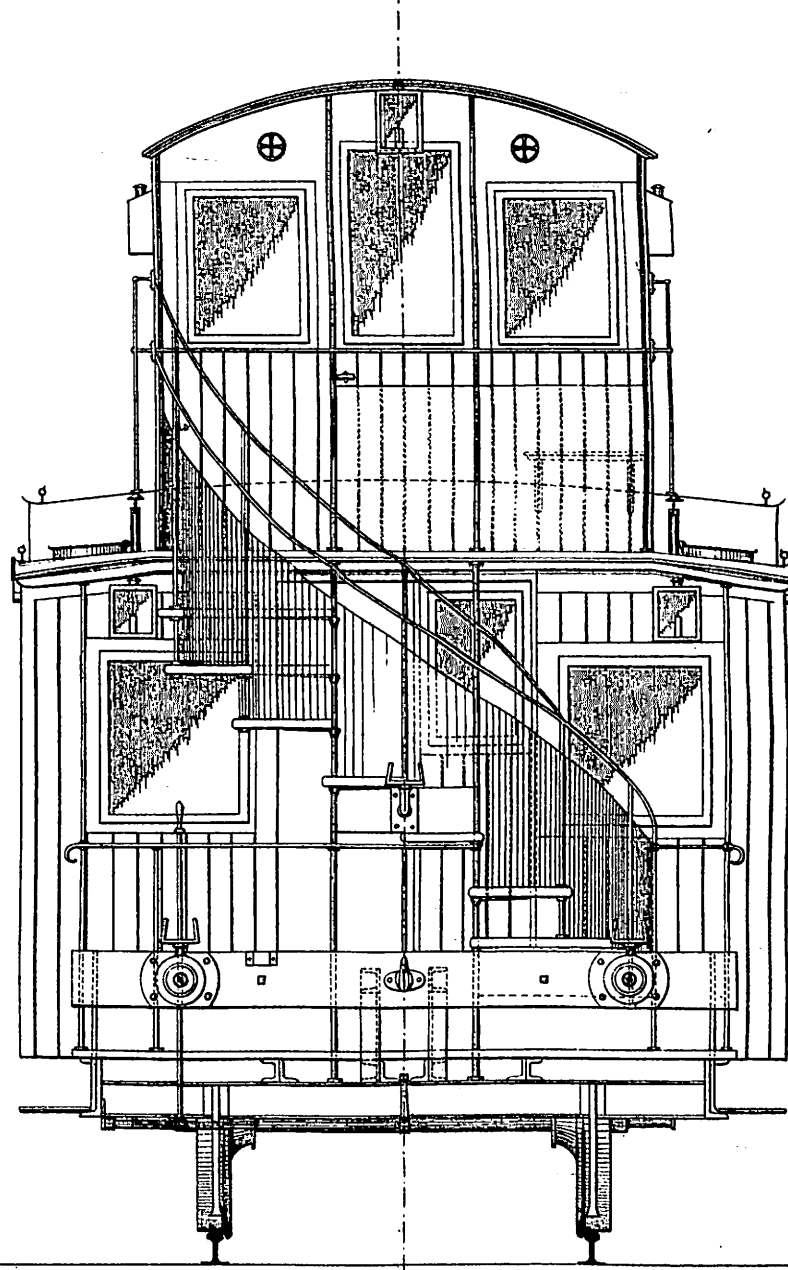
End-Ansicht.
