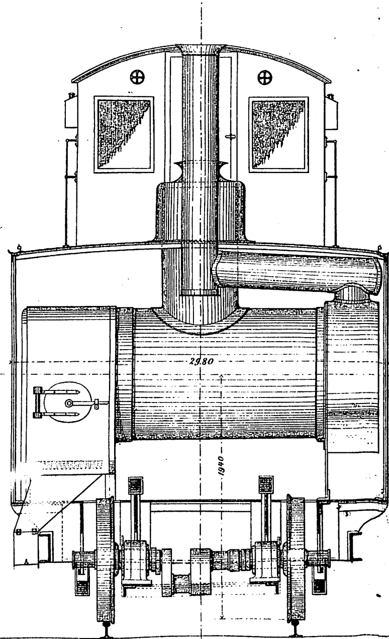
Schnitt AB.
