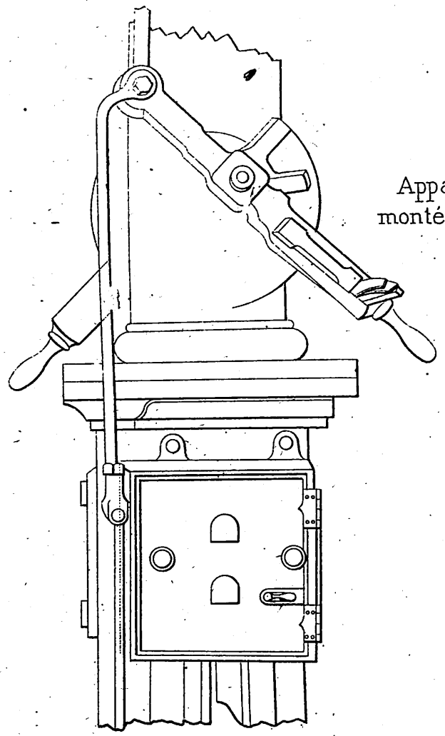
Fig. 3 Support de Block N° 3 pour Vignier vertical
