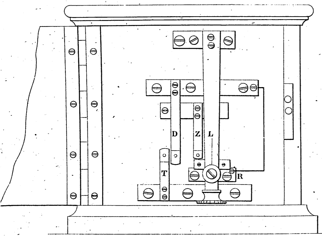
Bouton de Débloquage.
