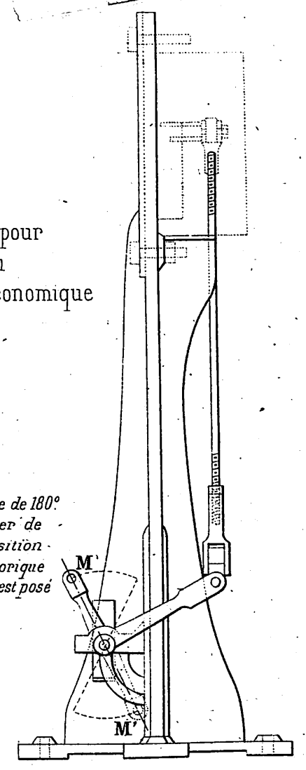
Fig. 4 Support de Block N° 3 pour Saxby
